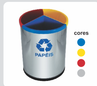
LIXEIRA MIX INOX COM 3 DIVISÕES PARA COLETA SELETIVA 420x315mm Capacidade: 26L cód.: MIX3i
